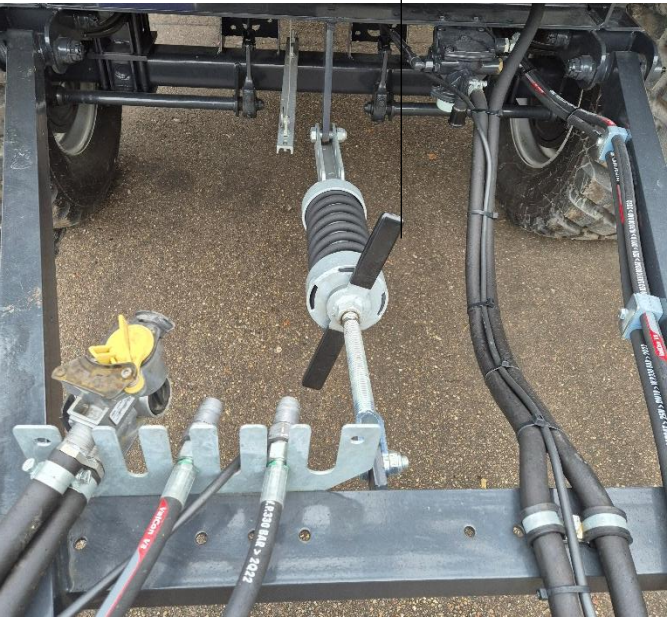
Stabile Deichselstütze und Schlauchhalterung (Serie)
